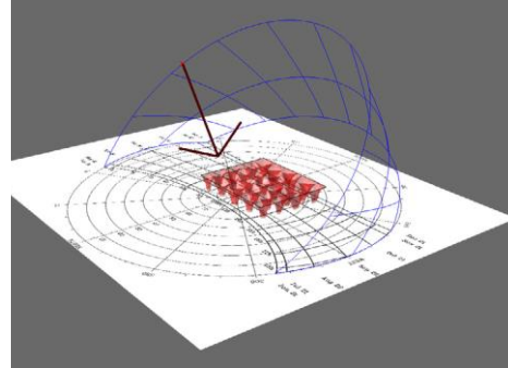
شكل (30) يوضح أنه بعد الانتهاء من تكرار الوحدة والوصول لتصميم السقف يتم عمل اختبارات عليه باستخدام برامج المحاكاه البيئة Sun-Shade Analysis لقياس نسبة التظليل واختيار أفضل مساحة للفتحات بالسقف وأفضل نسبة ميل
