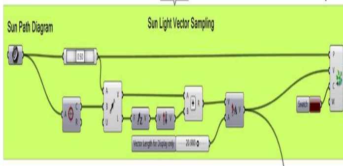
شكل (30) يوضح أنه بعد الانتهاء من تكرار الوحدة والوصول لتصميم السقف يتم عمل اختبارات عليه باستخدام برامج المحاكاه البيئة Sun-Shade Analysis لقياس نسبة التظليل واختيار أفضل مساحة للفتحات بالسقف وأفضل نسبة ميل
